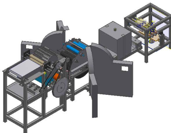
Figura 1: Vista de la máquina de transformación de fibra de alpaca (Elaboración propia)
