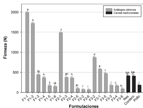
Figura 1: Valores de firmeza de 18 análogos de carne y carnes tradicionales
