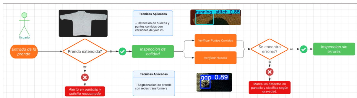
Figura 1: Pipeline de detección de huecos y puntos corridos en prendas de fibra de alpaca mediante visión computacional con YOLOv5.
