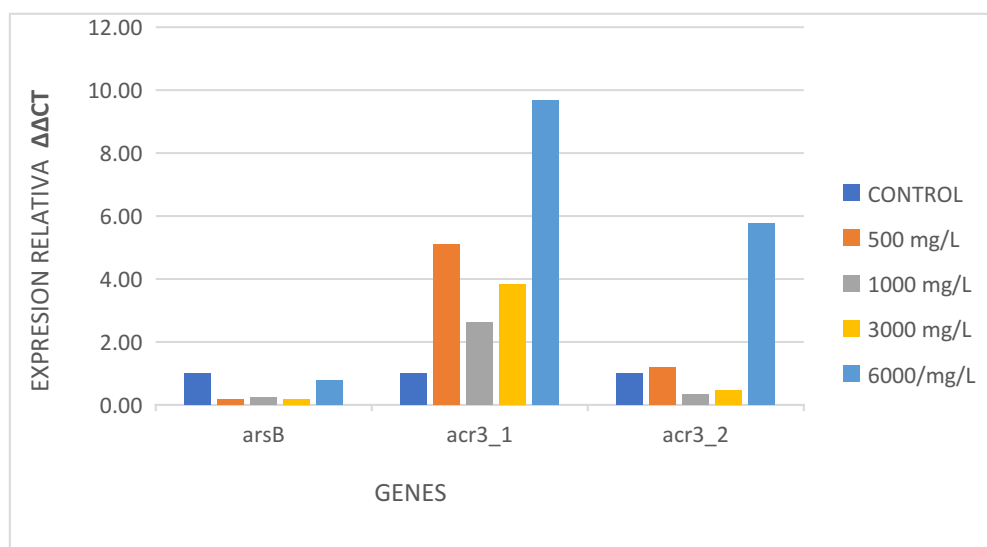
Figura 1: Expresión de las bombas de eflujo de Microbacterium algeriense , control (azul), 500 mg/L (anaranjado), 1000 mg/L (plomo), 3000 mg/L (amarillo) y 6000 mg/L (celeste).
