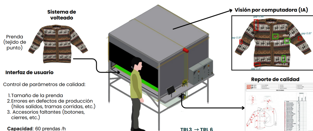
Figura 1: CAD de la máquina de control de calidad y reporte de inspección
