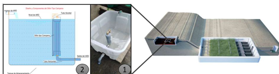
Figura 1: Diseño (1), componentes y funcionamiento (2) del sifón tipo campana.
