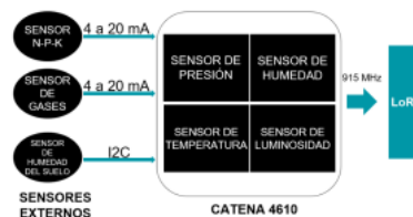
Fig6. Arquitectura Nodo-Sensor
