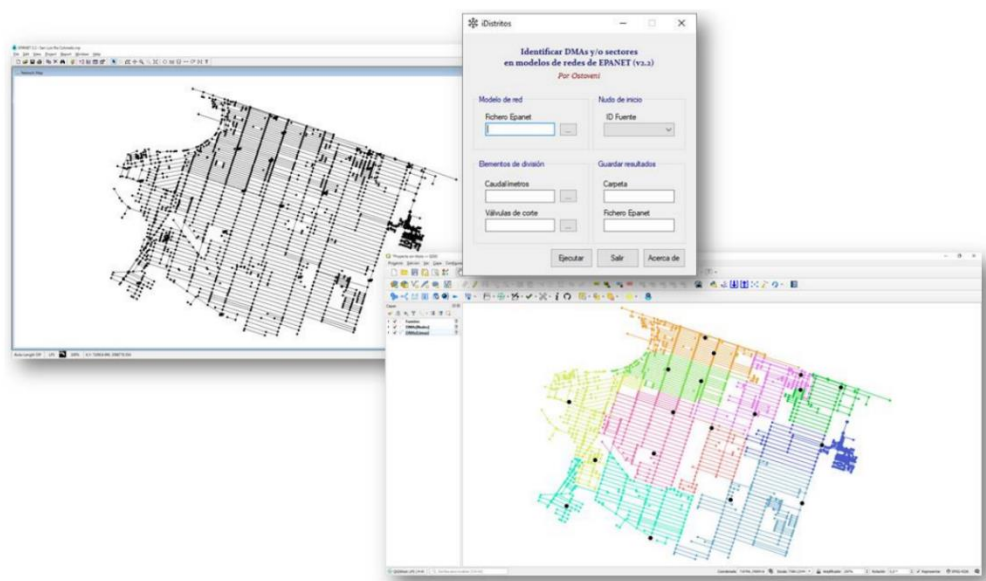
Figura 1. Sectorización de la red San Luis Rio Colorado (México).
